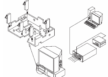
各式模具孔位及高度量測
