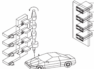
凸輪軸量測
