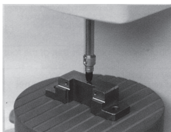
各式段差量測
