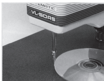
碟片厚度量測
