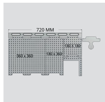
三次元量床定位托盤系統720
