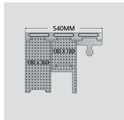
三次元量床定位托盤系統540
