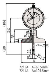
7213A A=63.5 mm 7214A A=101.6 mm
