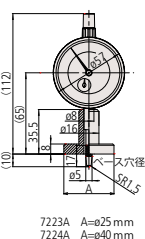
7223A A=25 mm 7224A A=40 mm
